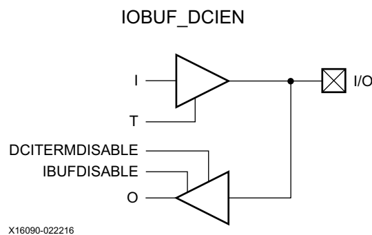
Figure 1-31: Input/Output Buffer DCI Enable Primitive (IOBUF_DCIEN)
